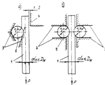
а — односрезное соединение; б — двухсрезное соединение; 1, 2 — стержни арматуры; 3 — сжимы; 4 — упор, препятствующий отгибу конца стержня 1; P — испытательная нагрузка
