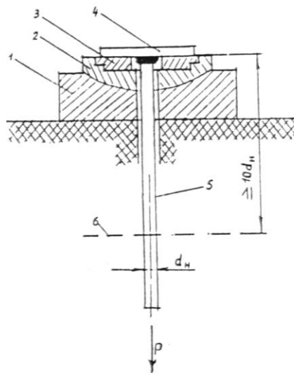
1 — сферическая опора; 2 — сферический вкладыш; 3 — сменное опорное кольцо; 4 — плоский элемент закладного изделия; 5 — анкерный стержень; 6 — граница закрепления в захвате разрывной машины; d_n — номинальный диаметр анкерного стержня; P — испытательная нагрузка
